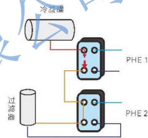
板式换热器在冷凝液净化中的应用
