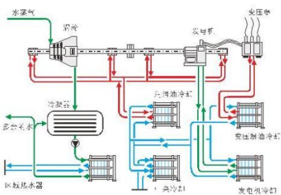
用于发电厂应用的 PHE
