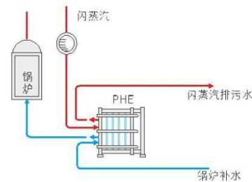
板式换热器在热回收中的应用
