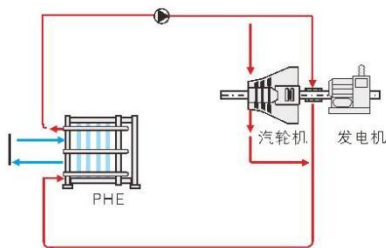
板式换热器在汽轮机润滑油冷却中的应用
