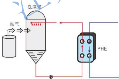
板式换热器在洗涤塔排水热回收中的应用
